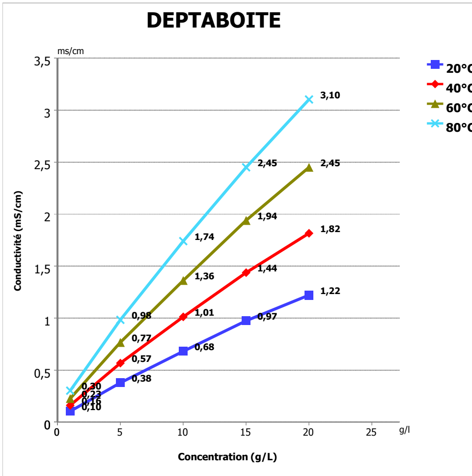
Courbe de conductivité
